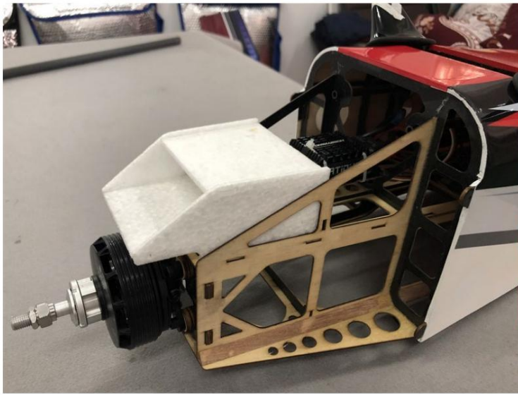
Capot d'installation et accessoires
